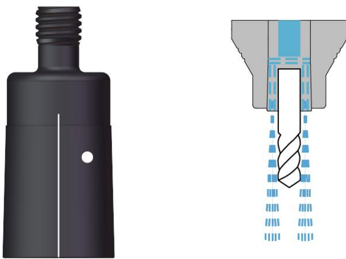
側面出水 + 固定銷
